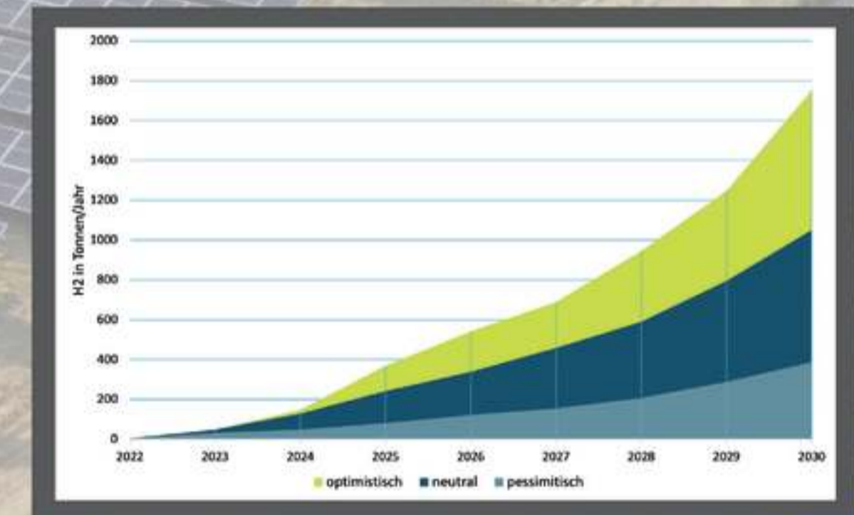
Hochlaufszenerario für die Nutzung von Wasserstoff in der Mobilität im Landkreis Wunsiedel i. Fichtelgebirge
